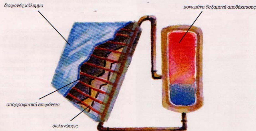
Τυπικό ενεργητικό ηλιακό σύστημα
